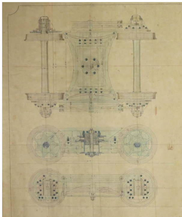
日本鉄道会社の蒸気機関車用先台車色彩図(部分)
