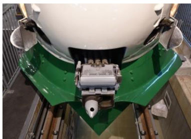
200系新幹線電車 連結器
